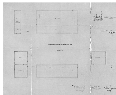
Plan de l'établissement de MM. Page frères au Valdoie (Haut-Rhin) [plan-masse]. Phot. Jérôme Mongreville IVR43_20019000028V
