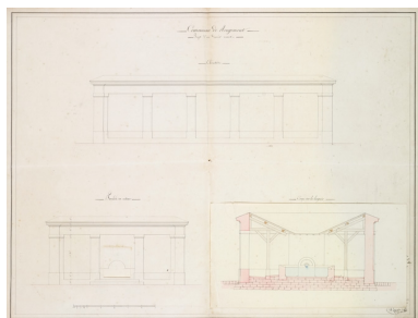
Commune de Rougemont. Projet d'un lavoir couvert. Façade en retour. Coupe sur la largeur. 1831. Phot. Jérôme Mongreville, Autr. César Convers IVR43_20102500567NUC2A
