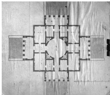
Plan du rez-de-chaussée logis carré avec rotonde centrale et quatre peristyles [plan de la villa Rotonda à Vicence ?]. Phot. Yves Sancey IVR43_19923901085X
