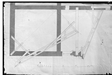
Détail des demi-fermes de la charpente. Phot. Yves Sancey IVR43_19923901088X
