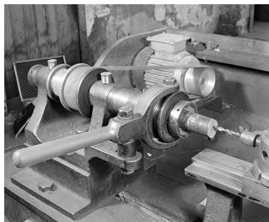
Détail du tour de gauche avec son moteur (atelier principal). Phot. Jérôme Mongreville IVR43_20022500626X
