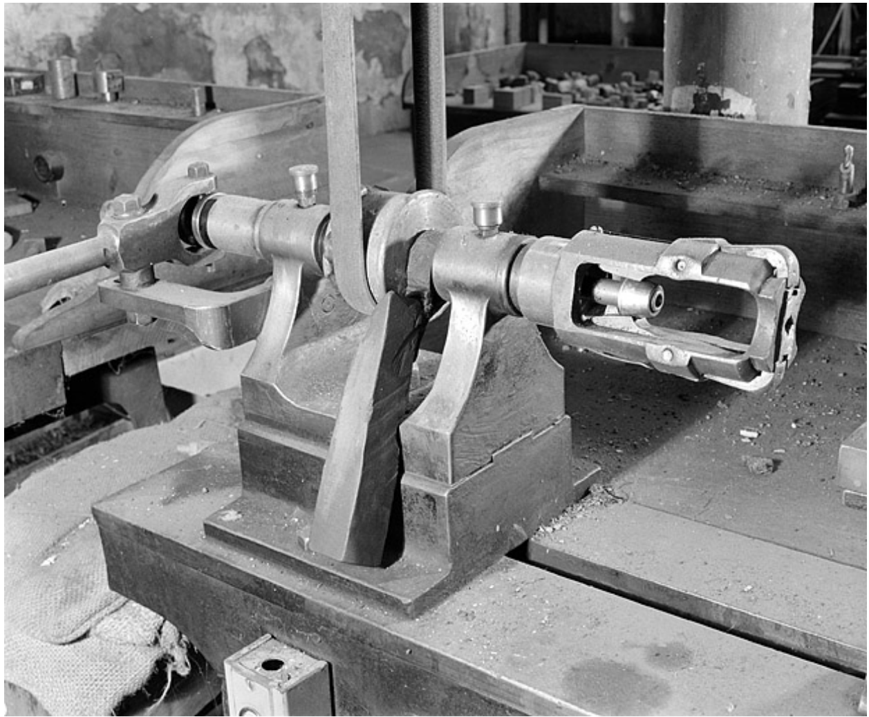
Tour central (atelier principal) : à gauche, la manette qui dessert les mâchoires.
