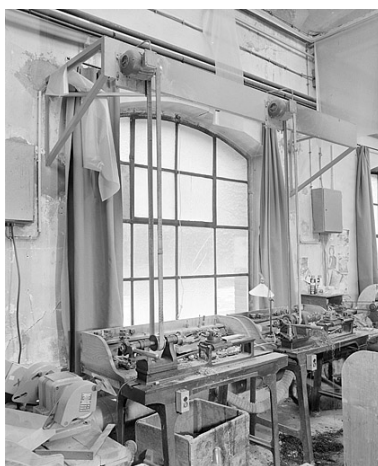
Vue d'ensemble de deux tours de l'atelier de finissage (avec leur moteur). Phot. Jérôme Mongreville IVR43_20022500475X
