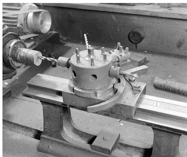
Détail du barillet du tour de gauche (atelier principal). Phot. Jérôme Mongreville IVR43_20022500627X
