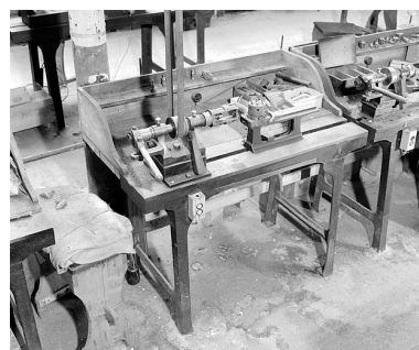
Vue d'ensemble rapprochée du tour central (atelier principal). Phot. Jérôme Mongreville IVR43_20022500631X
