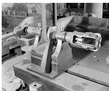
Tour central (atelier principal) : à gauche, la manette qui dessert les mâchoires. Phot. Jérôme Mongreville IVR43_20022500632X
