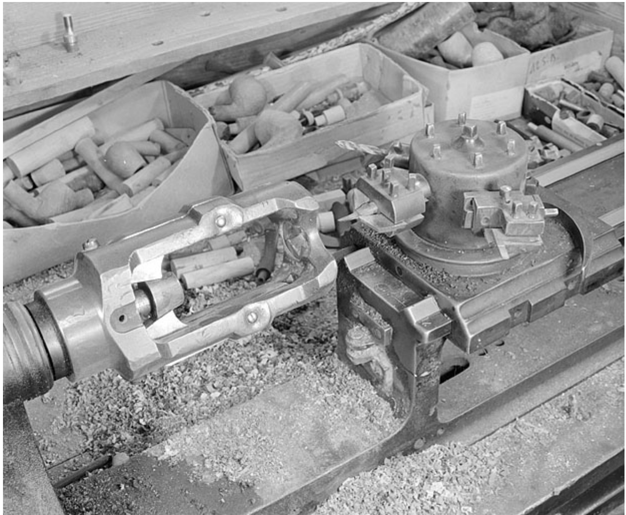
Tour (atelier de finissage). Les mâchoires et le revolver alignés.
