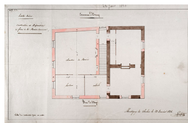
Proposition de Loiselot pour la construction de la maison commune : plan de l'étage. Phot. Jérôme Mongreville, Autr. Claude Loiselot
