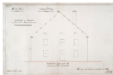
Proposition de Loiselot pour la construction de la maison commune : élévation de la façade côté sud. Phot. Jérôme Mongreville, Autr. Claude Loiselot IVR43_20167000918NUC4A
