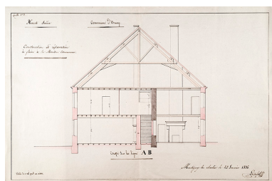
Proposition de Loiselot pour la construction de la maison commune : coupe. Phot. Jérôme Mongreville, Autr. Claude Loiselot IVR43_20167000916NUC4A
