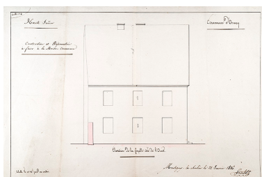
Proposition de Loiselot pour la construction de la maison commune : élévation de la façade côté ouest. Phot. Jérôme Mongreville, Autr. Claude Loiselot IVR43_20167000917NUC4A
