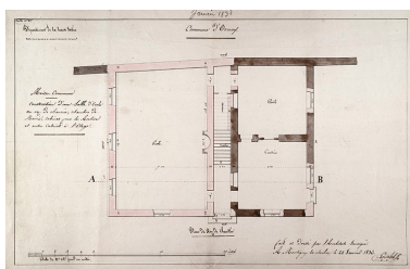
Proposition de Loiselot pour la construction de la maison commune : plan du rez-de-chaussée. Phot. Jérôme Mongreville, Autr. Claude Loiselot
