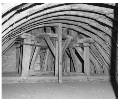
Charpente du comble et beffroi Phot. Michel Thierry IVR26_19852101217X
