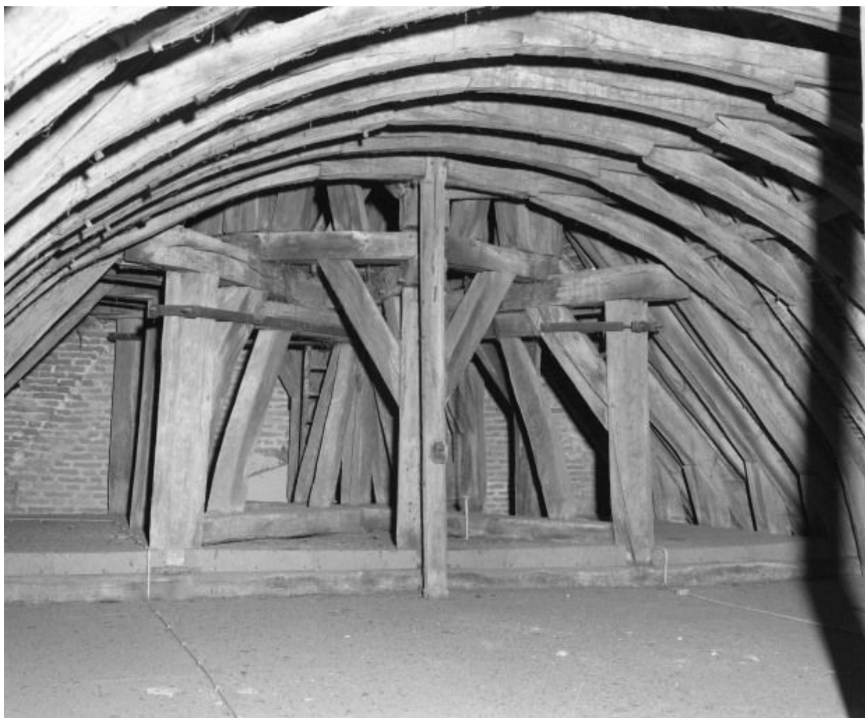
Charpente du comble et beffroi
