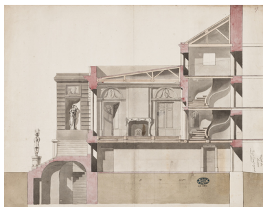
[Triplot des Barres ou ancienne Comédie. Projet de corps d'entrée (non réalisé) : coupe partielle]. S.d. [décennie 1770 ?]. Phot. Pierre-Marie Barbe-Richaud, Autr. auteur inconnu IVR26_20222100812NUC4A
