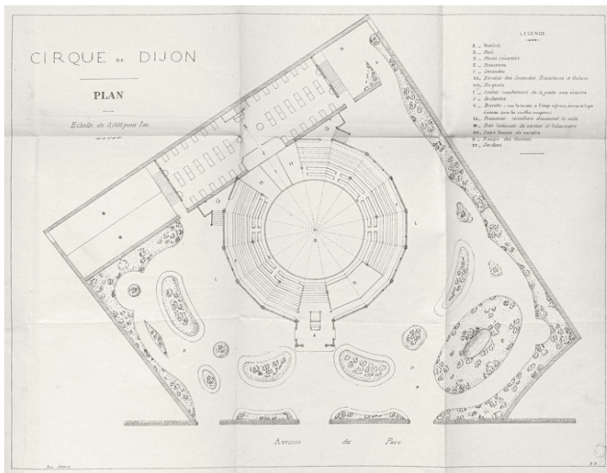
Cirque de Dijon [Cirque-Théâtre d'Eté, 4 cours du Général de Gaulle]. Plan. S.d. [1869].
