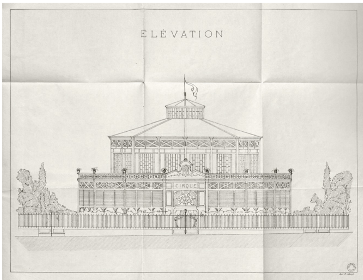
Cirque de Dijon [Cirque-Théâtre d'Été, 4 cours du Général de Gaulle]. Elévation. S.d. [1869].
