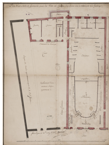
Plan d'une salle de spectacles pour la ville de Chalon sur Saône avec le bâtiment du concierge. 30 mai 1746. Phot. Pierre-Marie Barbe-Richaud, Autr. Charles-Elie Le Jolivet IVR26_20222100815NUC4A
