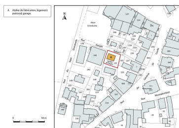
Plan-masse et de situation. Extrait du plan cadastral, 2015, section AK. Dess. Mathias Papigny IVR43_20152502326NUDA
