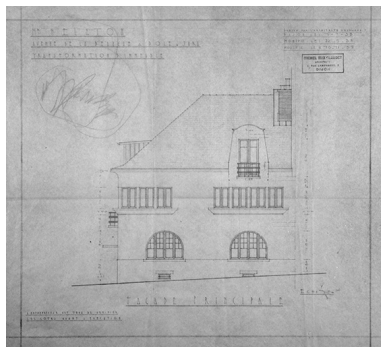
M. Nélaton [...] Transformation d'immeuble. Façade principale. Phot. Jérôme Mongreville, Autr. Michel-Max (architecte) Claudet IVR43_19893900212X
