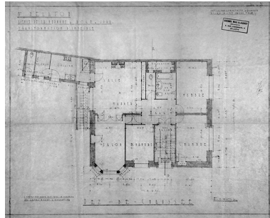
M. Nélaton [...] Transformation d'immeuble. Rez-de-chaussée. Phot. Jérôme Mongreville, Autr. Michel-Max (architecte) Claudet IVR43_19893900210X
