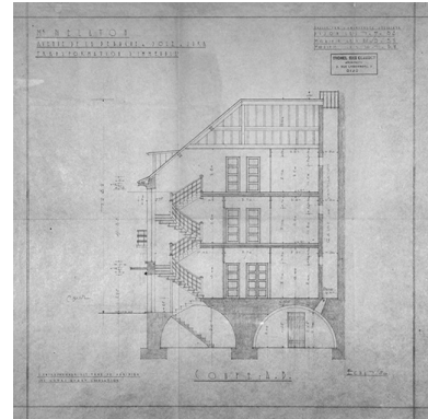
M. Nélaton [...] Transformation d'immeuble. Coupe A.B. (coupe transversale). Phot. Jérôme Mongreville, Autr. Michel-Max (architecte) Claudet IVR43_19893900211X
