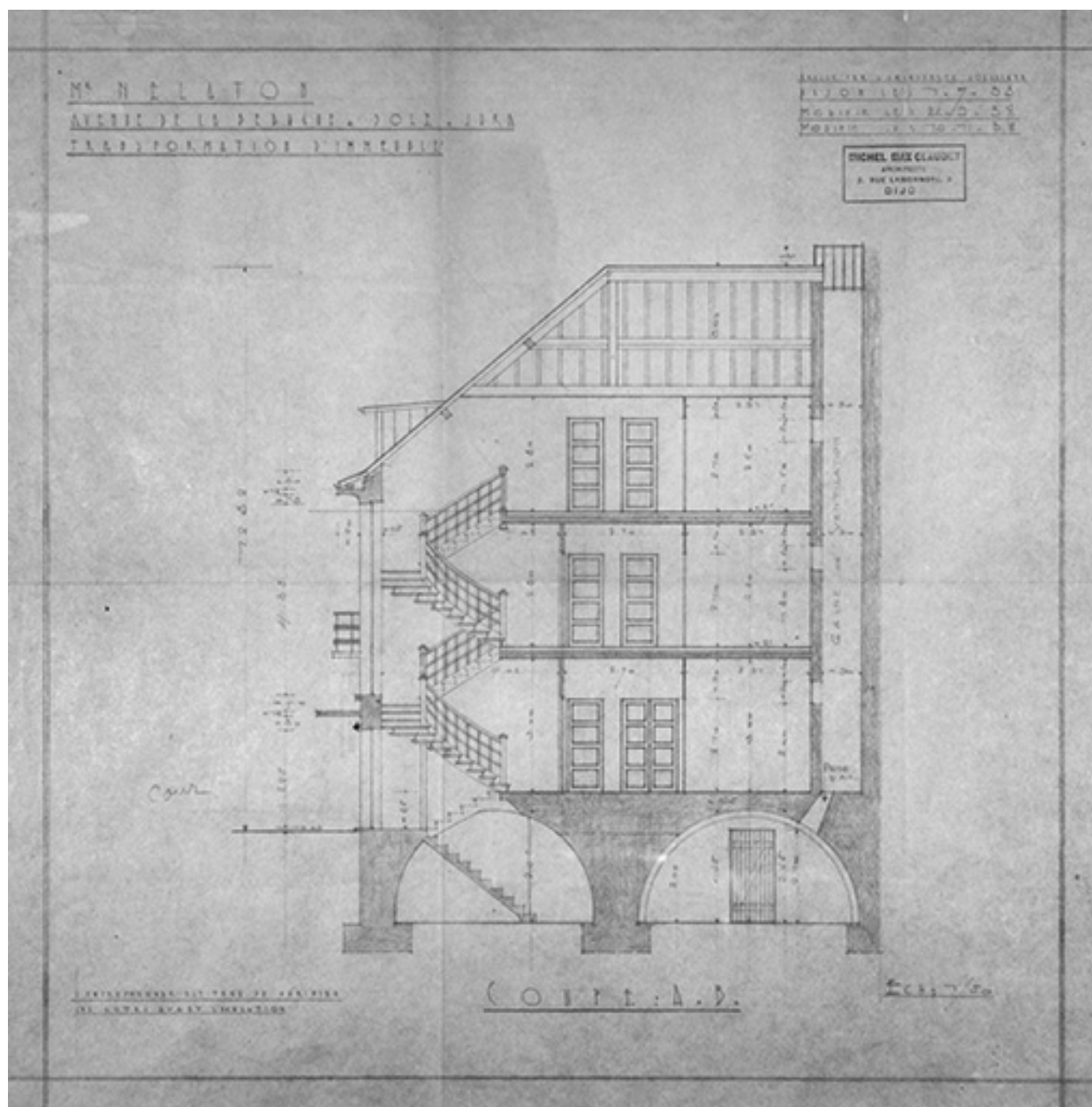
M. Nélaton [...] Transformation d'immeuble. Coupe A.B. (coupe transversale).
