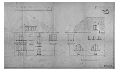
M. Nélaton [...] Transformation d'immeuble. Façade sur cour et Façade sur rue [projet non réalisé]. Phot. Jérôme Mongreville, Autr. Michel-Max (architecte) Claudet IVR43_19893900214X
