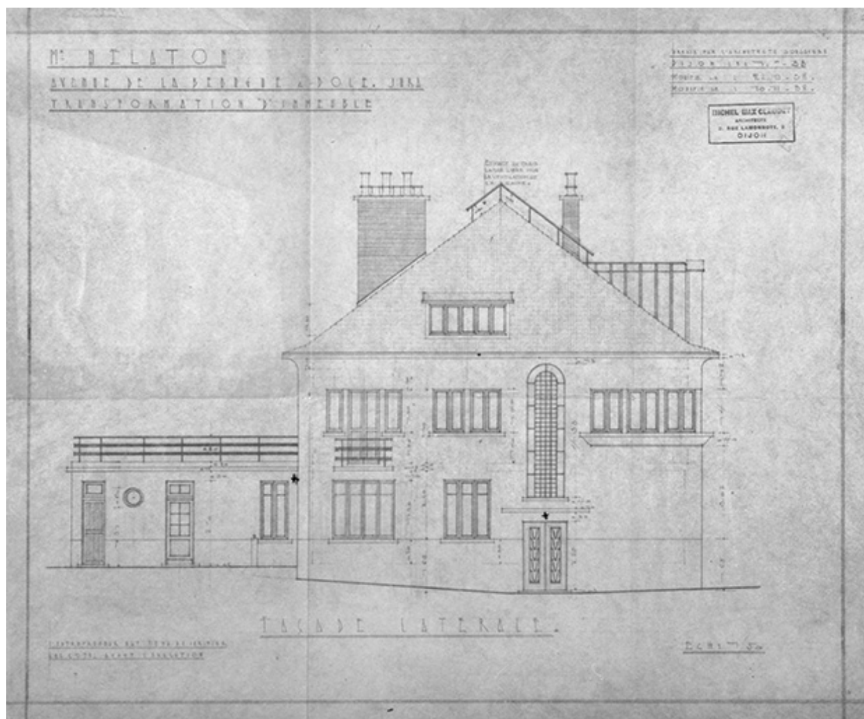
M. Nélaton [...] Transformation d'immeuble. Façade latérale.
