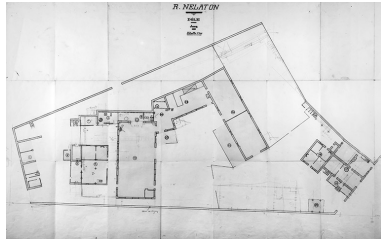
R. Nélaton. Dole. Jura. Plan de distribution de l'usine et du logement patronal. Phot. Jérôme Mongreville IVR43_19893900209X
