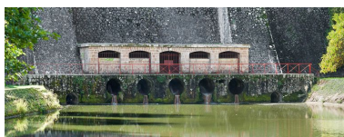
Vue extérieure de la chambre des robinets située en contrebas de la digue. Phot. Pierre-Marie Barbe-Richaud IVR26_20112103644NUC4AQ
