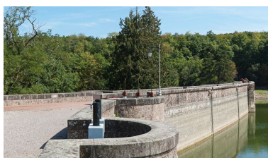
Vue de la digue du réservoir. Phot. Pierre-Marie Barbe-Richaud IVR26_20112103621NUC4AQ
