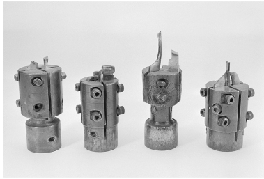
Détail de quatre outils de coupe. Phot. Jérôme Mongreville IVR43_20022500955X
