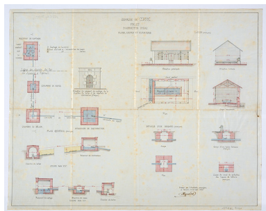
Commune de Corre. Projet d'adduction d'eau. [plans, coupes, élévations.] 1910 Phot. Sonia Dourlot IVR43_20167000087NUC4A
