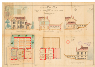
Commune de Nods. Projet de construction d'un chalet-modèle. Plans, coupe et élévations, 1906. Phot. Sonia Dourlot IVR43_20152500542NUC4A
