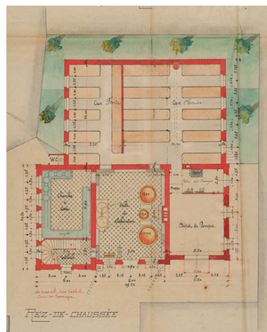
Projet de construction d'un chalet-modèle. Plan du rez-de-chaussée, 1906. Phot. Sonia Dourlot IVR43_20152500506NUC4A
