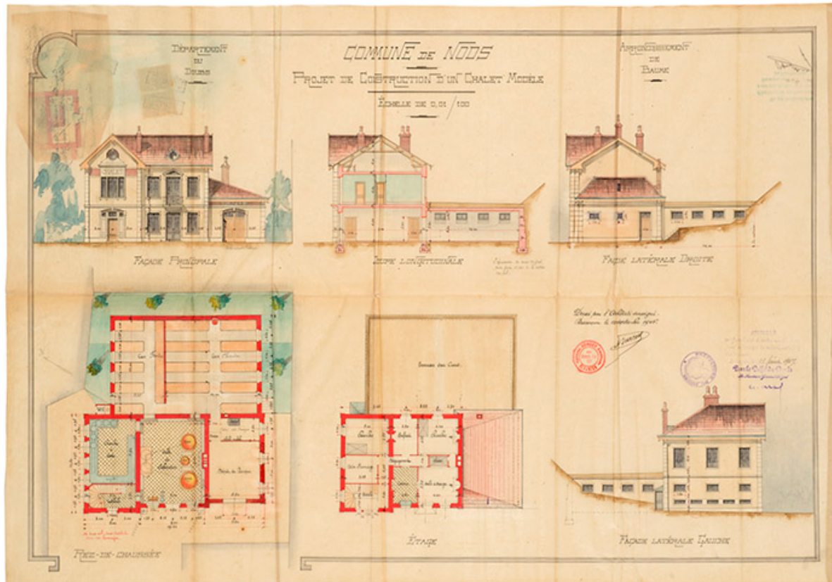
Commune de Nods. Projet de construction d'un chalet-modèle. Plans, coupe et élévations, 1906.
