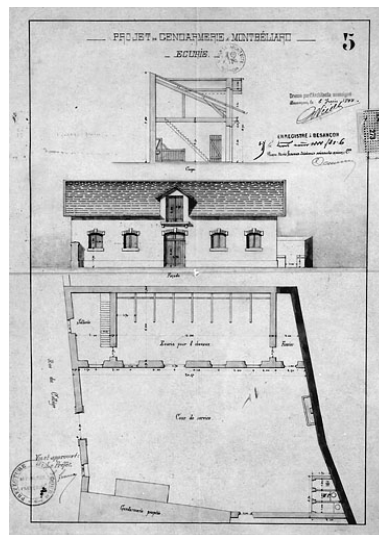
Projet de Gendarmerie à Montbéliard. Ecuries, 1888. Phot. Jérôme Mongreville, Phot. Gustave Vieille IVR43_19872500211X
