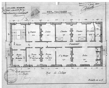
Projet de Gendarmerie à Montbéliard. Plan du rez-de-chaussée, 1888. Phot. Jérôme Mongreville, Phot. Gustave Vieille IVR43_19872500209X
