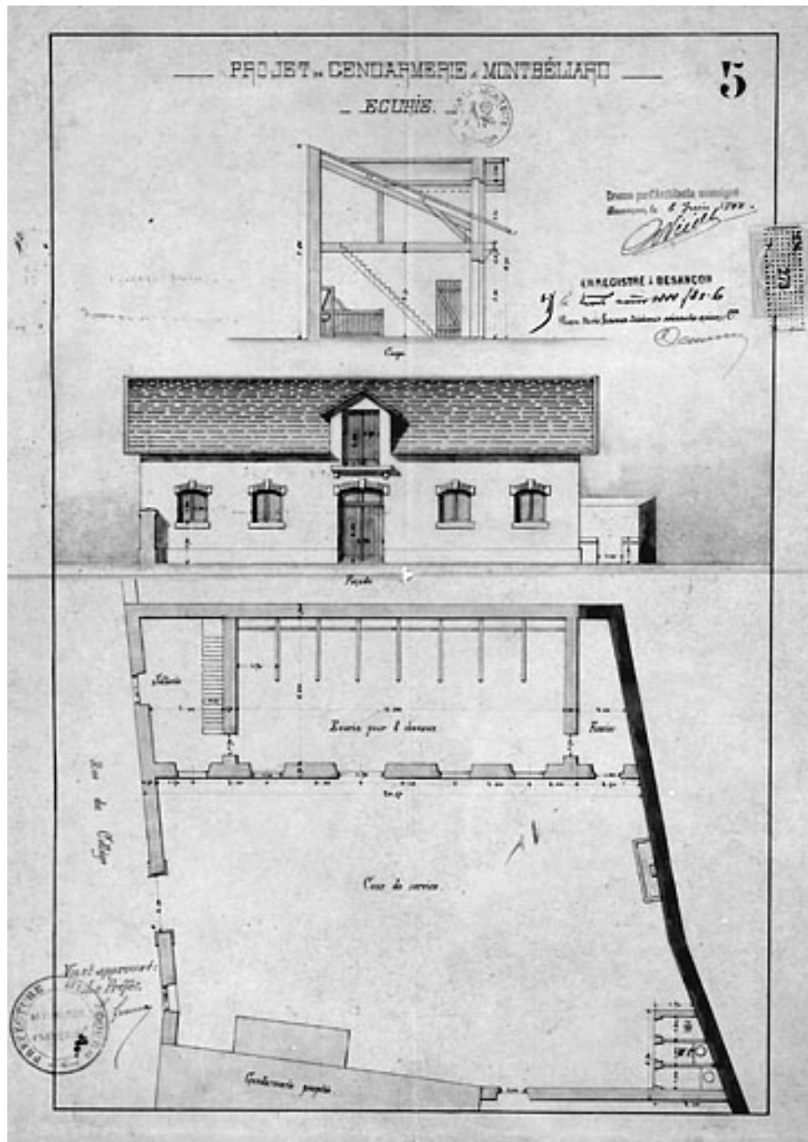
Projet de Gendarmerie à Montbéliard. Ecuries, 1888.
