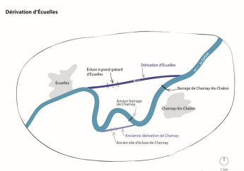
Plan schématique de la dérivation d'Écuellles, échelle 1 / 2 000e. Dess. Aline Thomas IVR26_20227100070NUDA
