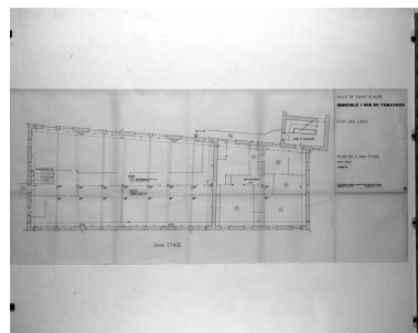
Immeuble 1 rue du Tomachon. Etat des lieux. Plan du 2ème étage.
