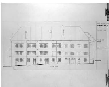
Immeuble 1 rue du Tomachon. Etat des lieux. Façade nord.
