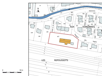
Plan-masse et de situation. Dess. Mathias Papigny IVR43_20132502567NUDA
