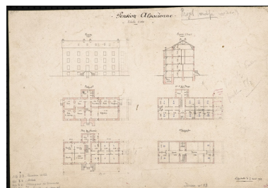
Pension alsacienne. Plans, coupes, élévation, échelle 1/250, Lafeschotte, 7 août 1923. Phot. Jérôme Mongreville, Autr. IVR43_20122501208NUC4A
