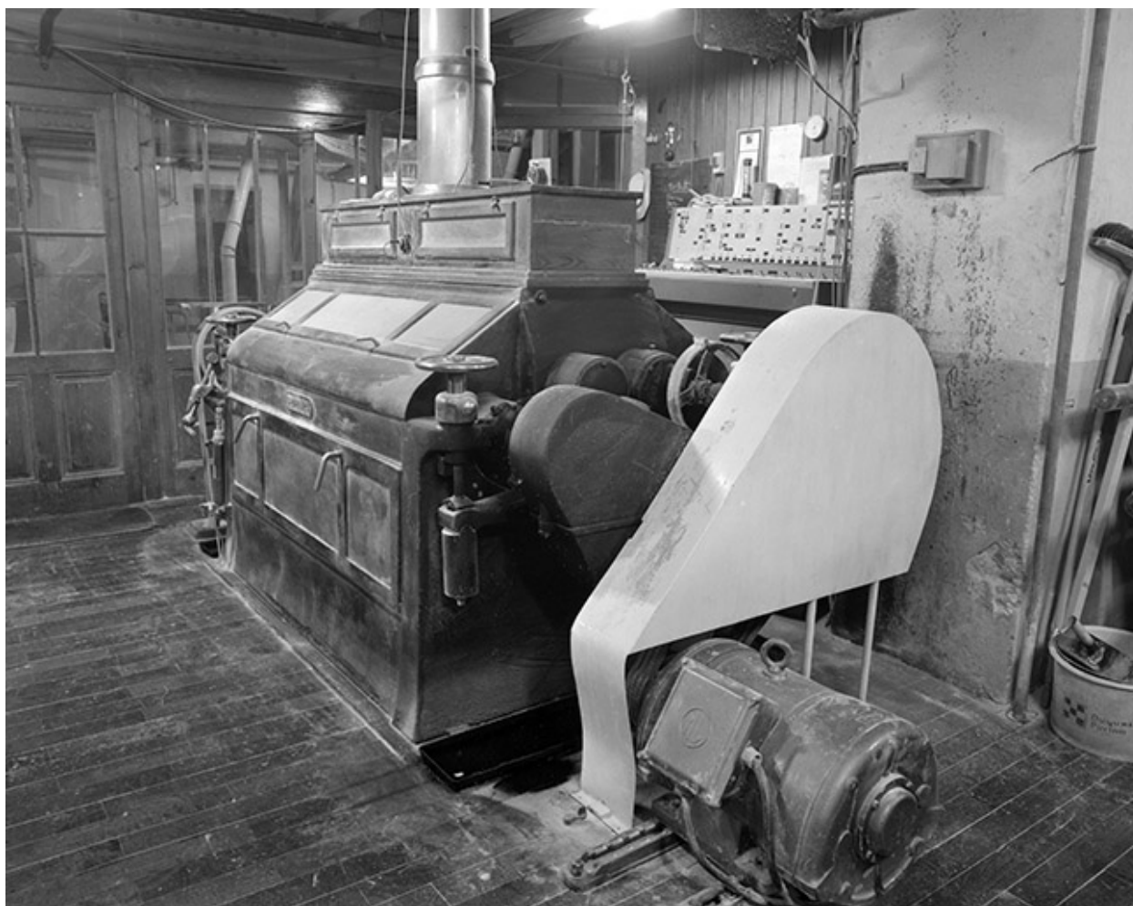
Appareil à cylindres Buhler.
