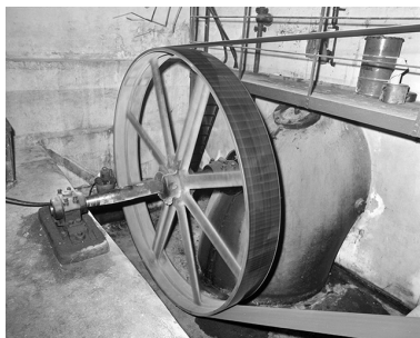
Volant de transmission de la turbine Francis. Phot. Jérôme Mongreville IVR43_19963900044X
