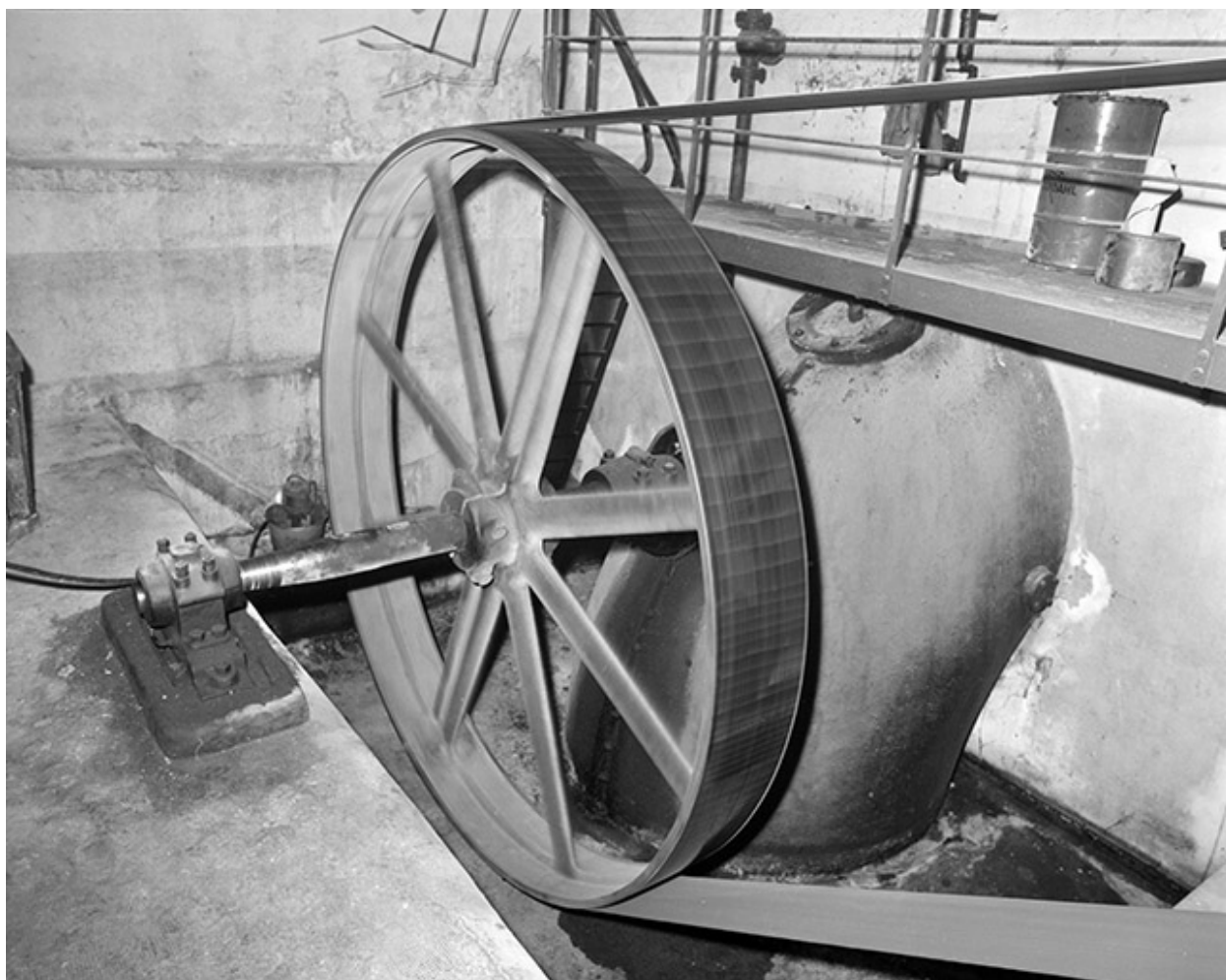
Volant de transmission de la turbine Francis.
