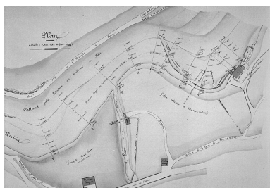
Usine hydraulique des fils de Louis Lahu négociants à Lavans [...] Plan. Phot. Jérôme Mongreville, Phot. Messin IVR43_19943900452X
