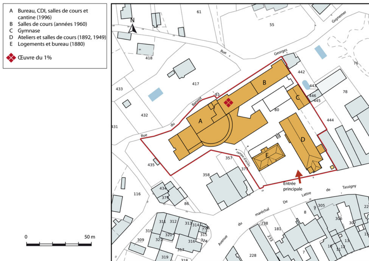
Plan-masse et de situation. Extrait du plan cadastral numérisé, section AL, échelle 1:1000.
