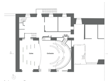
Projet de restauration : plan du rez-de-chaussée. D'après un plan de l'architecte Olivier Chanu, dessiné par M.P. en 2018. Dess. Aline Thomas, Autr. Olivier Chanu IVR26_20237100039NUDA
