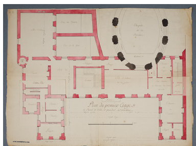
Plan du premier étage de l'hotel de ville et présidial de Salins (avec entresol), s.d. [vers 1720].
