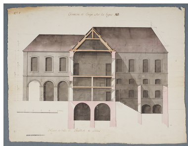
Hotel de ville et présidial de Salins. Elévation et coupe sur la ligne AB, s.d. [vers 1720].
