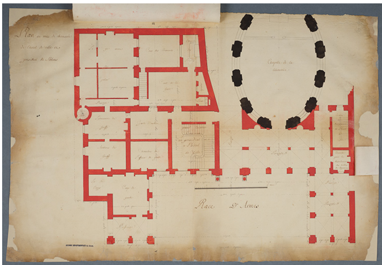
Plan du rez de chaussée de l'hôtel de ville et du présidial de Salins, s.d. [vers 1720].
