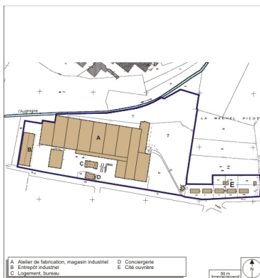
Plan-masse et de situation. Extrait du plan cadastral, 2008, section AD, 1:1250 réduit à 1:2700. Source : Direction générale des Finances Publiques - Cadastre ; mise à jour : 2008. Dess. André Céréza IVR43_20087000198NUDA
