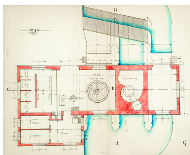
Usine électrique du Châtelot, plan, 1917. Phot. Jérôme Mongreville, Autr. auteur inconnu IVR43_20132500497NUC4A
