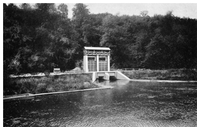
USINE DU CHATELOT : La prise d'eau.
