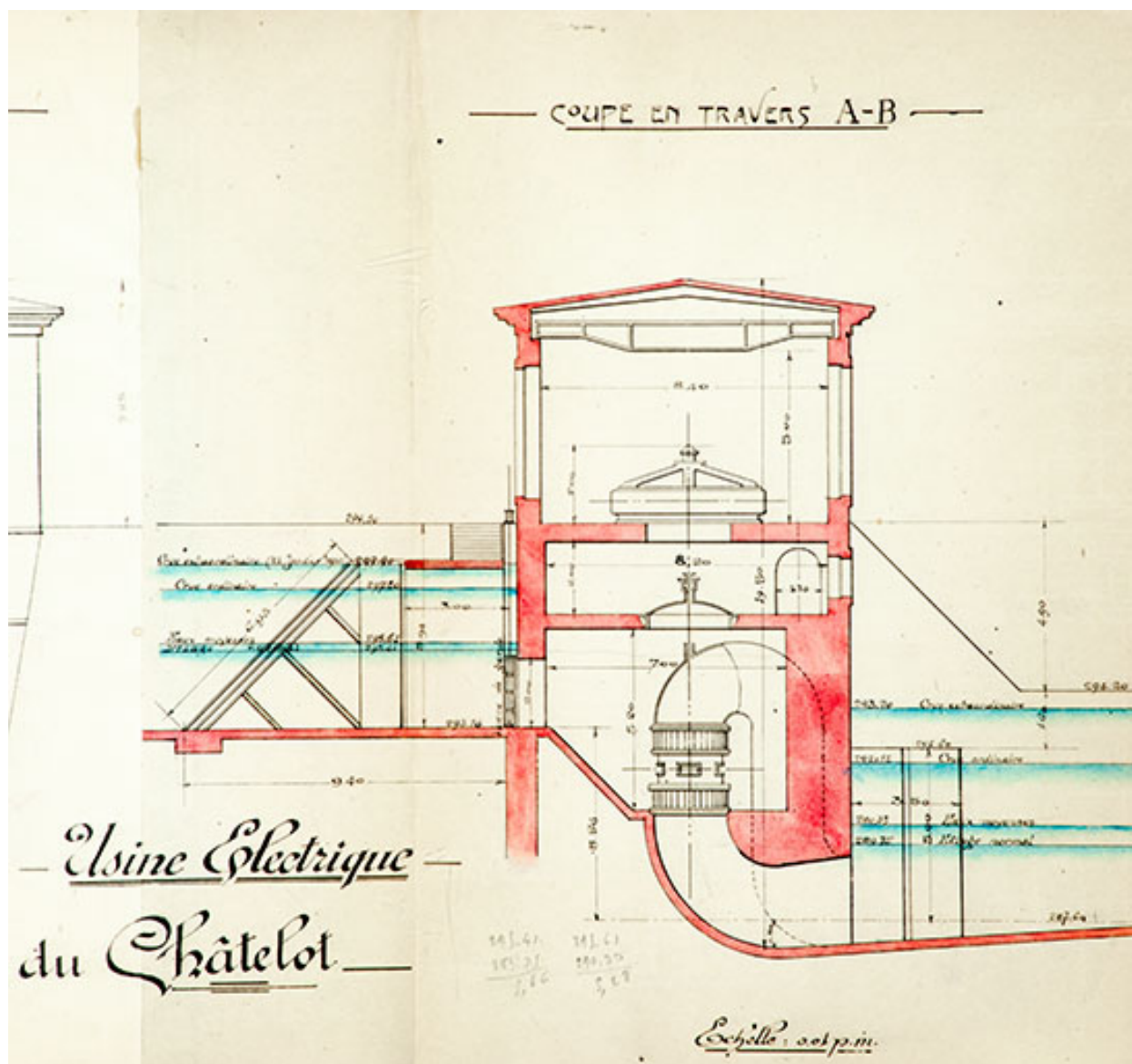
Usine électrique du Châtelot, coupe en travers, 1917.
