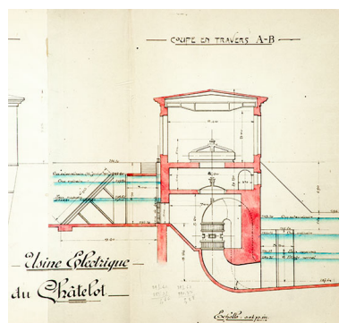
Usine électrique du Châtelot, coupe en travers, 1917. Phot. Jérôme Mongreville, Autr. auteur inconnu IVR43_20132500496NUC4A
