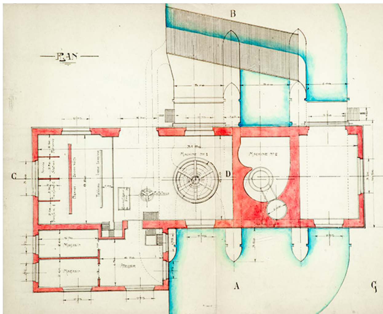
Usine électrique du Châtelot, plan, 1917.
