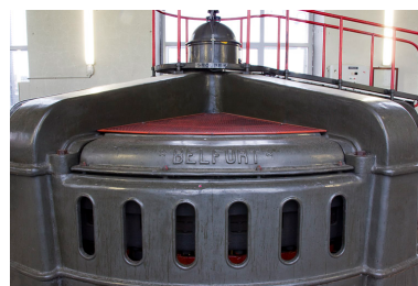
Détail d'un alternateur SACM. Phot. Yves Sancey IVR43_20122502062NUC2A
