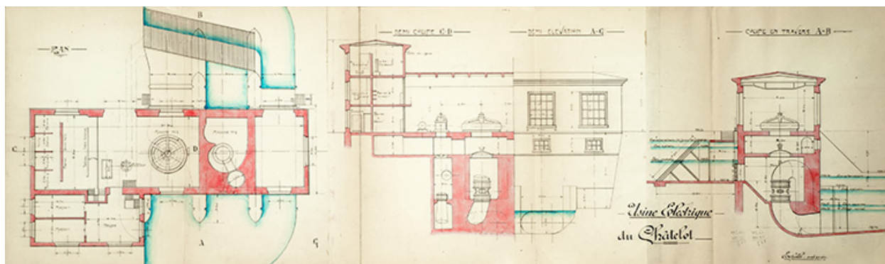
Usine électrique du Châtelot, plan, coupe, élévation, 1917.
