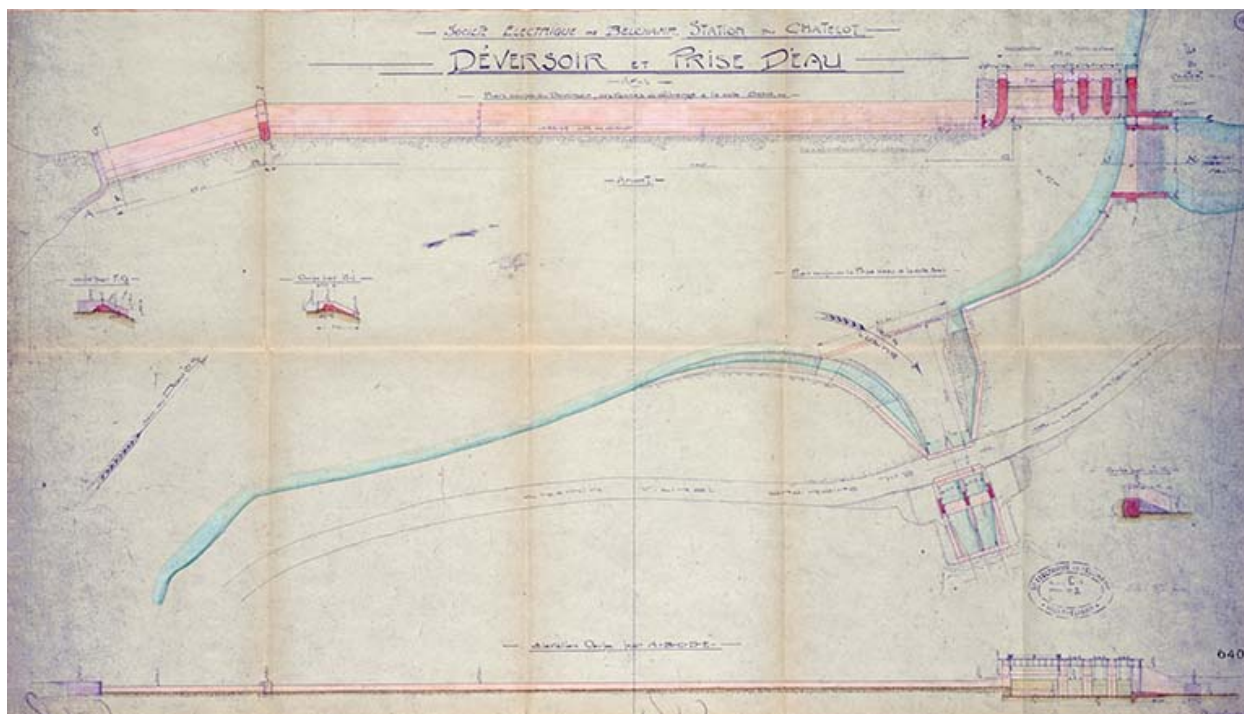
Société Electrique de Belchamp. Station du Chatelot. Déversoir et prise d'eau, pièce n° 6, 1934.
