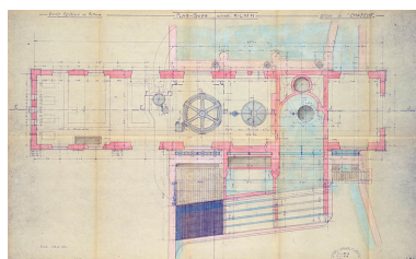
Société Electrique de Belchamp. Station du Chatelot. Plan-coupe de l'usine, pièce n° 9, 1934. Phot. Jérôme Mongreville, Autr. auteur inconnu IVR43_20132500486NUC4A
