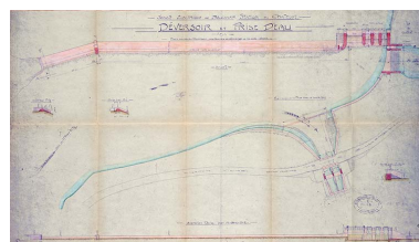
Société Electrique de Belchamp. Station du Chatelot. Déversoir et prise d'eau, pièce n° 6, 1934. Phot. Jérôme Mongreville, Autr. auteur inconnu IVR43_20132500488NUC4A
