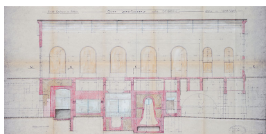
Société Electrique de Belchamp. Station du Chatelot. Coupe longitudinale de l'usine, pièce n° 11, 1934. Phot. Jérôme Mongreville, Autr. auteur inconnu IVR43_20132500485NUC4A
