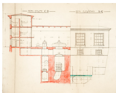
Usine électrique du Châtelot, demi- coupe et demi-élévation, 1917. Phot. Jérôme Mongreville, Autr. auteur inconnu IVR43_20132500495NUC4A
