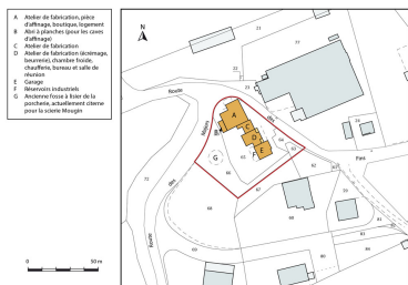
Plan-masse et de situation. Dess. Mathias Papigny IVR43_20162501484NUDA
