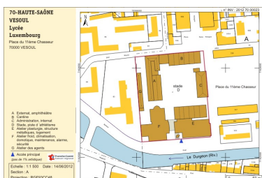
Plan-masse et de situation. Extrait du plan cadastral numérisé, section A, échelle 1:1500. Dess. André Céréza IVR43_20127000023NUDA
