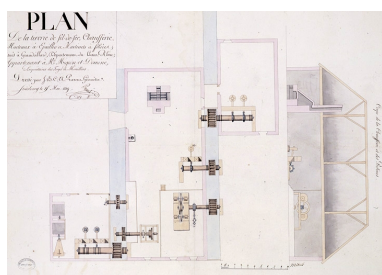
Plan de la tirerie de fil-de-fer, chaufferie, marteaux à épauiller et martinets à filières [...] [coupe longitudinale et plan au sol]. Phot. Jérôme Mongreville, Autr. NEPASUTILISERParent (géomètre) IVR43_20019000042VA
