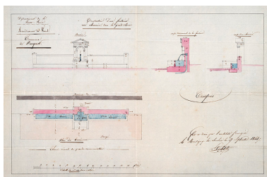
Projet de construction d'une fontaine par l'architecte Claude Loiselot, 1844. Phot. Jérôme Mongreville, Autr. Claude Loiselot IVR43_20187000250NUC4A
