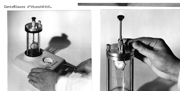
Société Yema : contrôleur d'étanchéité, photogr., s.d. [vers 1970]. IVR43_20212500119NUC1A
