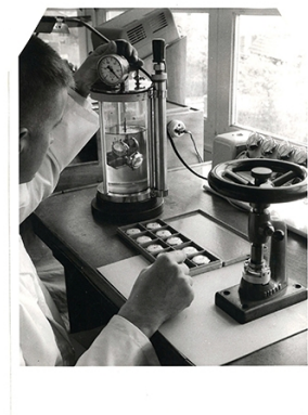
Société Yema : contrôle d'étanchéité, photogr., s.d. [vers 1970]. IVR43_20212500113NUC1A
