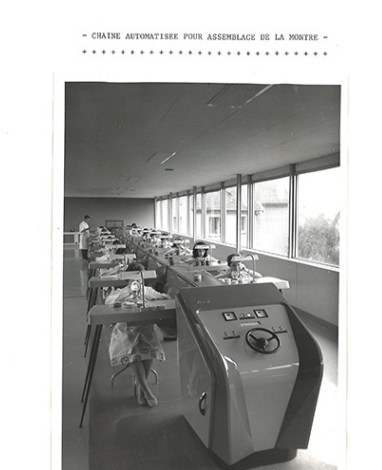
Société Yema : chaîne automatique d'assemblage des montres, photogr., s.d. [vers 1970]. IVR43_20212500117NUC1A
