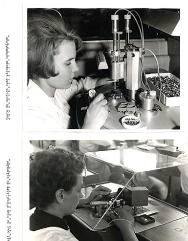
Société Yema : Projecteur pour contrôle et retouche des échappements, et assemblage par vissage électrique, photogr., s.d. [vers 1970]. IVR43_20212500115NUC2A
