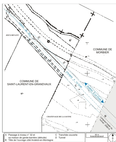
Plan-masse et de situation de la partie côté Andelot-en-Montagne (nord-ouest). Montage d'extraits du plan cadastral informatisé, 2006, Morbier, section BR (1:2000),
