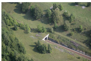
Vue aérienne rapprochée de la tête côté La Cluse, depuis le sud. Phot. Jean-Pierre Bévalot IVR43_20053900965NUCA
