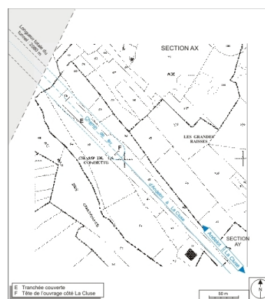
Plan-masse et de situation de la partie côté La Cluse (sud-est). Extrait du plan cadastral informatisé, 2007, section AX, échelle 1:2500. Dess. André Céréza IVR43_20073900300NUDA
