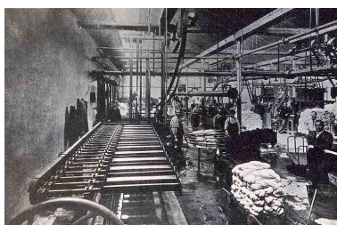
Atelier de teinturerie. Phot. Jérôme Mongreville IVR43_20067000232NUCA
