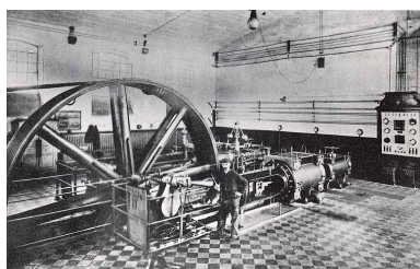
Machine à vapeur. Phot. Jérôme Mongreville IVR43_20067000218NUCA
