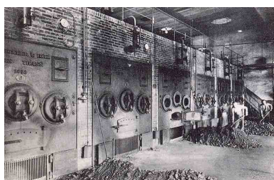
Chaufferie (chaudières Scheidecker et Kohl). Phot. Jérôme Mongreville IVR43_20067000207NUCA
