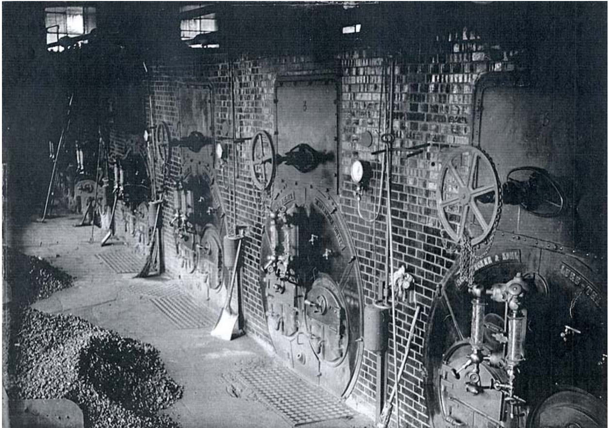
Chaudières à charbon Scheidecker et Kohl.
