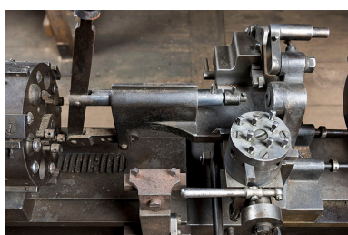
Vue plongeante sur la partie travaillante. Tourelle revolver au premier plan. Phot. Sonia Dourlot IVR43_20172500078NUC4A
