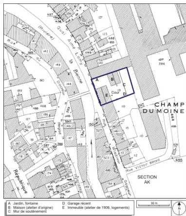
Plan-masse et de situation. Extrait du plan cadastral, 1980, section AI, échelle 1:1000. Dess. André Céréza IVR43_20093900310NUDA
