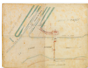
Exhaussement des barrages de Charnay et de Verdun-sur-le-Doubs. Barrage de Charnay. Plan des lieux et profils. 25 février 1880. Phot. Thierry Kuntz IVR26_20197100701NUC4A
