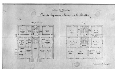
Salines de Montaigu. Plans des logements et bureaux de la Direction. Phot. Jérôme Mongreville IVR43_19963900204X
