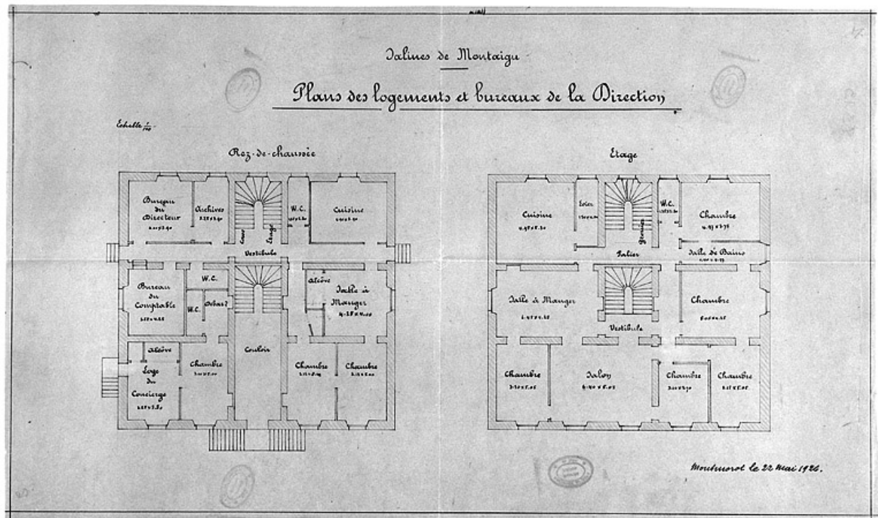
Salines de Montaigu. Plans des logements et bureaux de la Direction.
