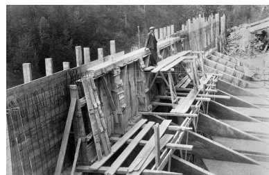
Construction du bassin de retenue. Phot. Jérôme Mongreville IVR43_19913900244X
