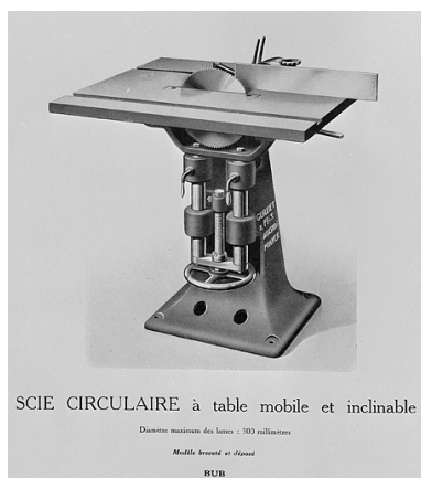
Scie circulaire à table mobile et inclinable. Phot. Yves Sancey IVR43_20022500919X
