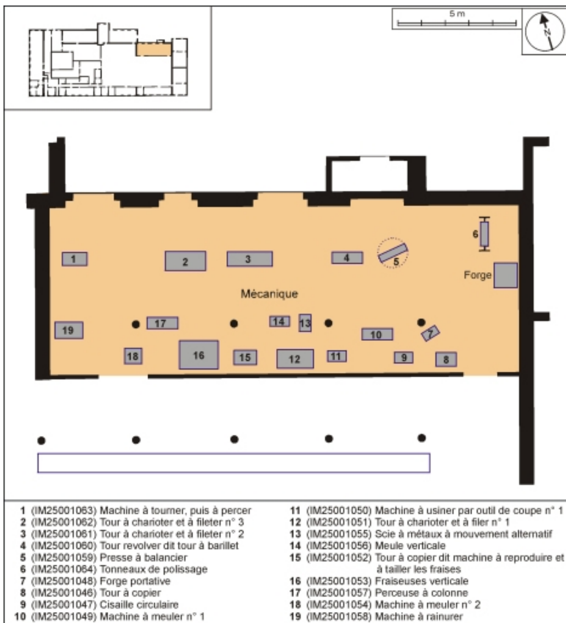
Plan de localisation des machines de l'atelier de mécanique.
