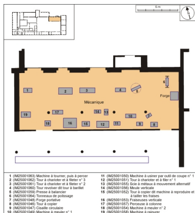
Plan de localisation des machines de l'atelier de mécanique. Dess. André Céréza IVR43_20022501339NUDA
