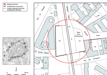
Plan masse et de situation. Extrait du plan cadastral, 2026, 1/1000. Dess. Aline Thomas IVR43_20262100201NUDA
