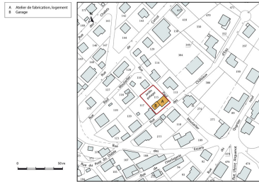
Plan-masse et de situation. Dess. Mathias Papigny IVR43_20162501529NUDA
