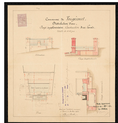
Distribution en eau, construction d'un lavoir. [plan] 1901 Phot. Sonia Dourlot IVR43_20167000107NUC4A
