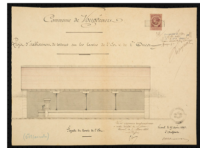
Projet d'établissement de toitures sur les lavoirs de l'est et de l'ouest. [Élévation] 1887 Phot. Sonia Dourlot IVR43_20167000109NUC4A
