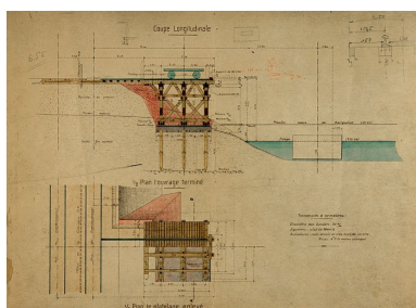
Besançon, port des Près-de-Vaux : exploitation militaire du Canal du Rhône au Rhin. Installation de transbordement au port des Près-de-Vaux, à Besançon. Projet définitif. Dessins de l'appontement [détail : plans et coupe longitudinale], 1918.
