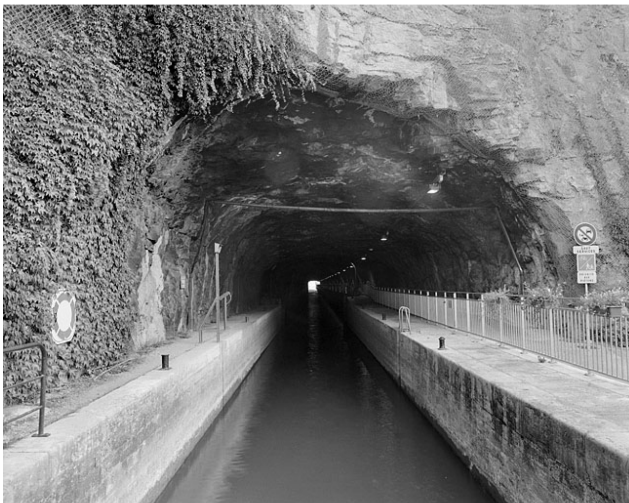
Besançon, site d'écluse n° 50 N de Tarragnoz : sas de l'écluse, depuis l'aval.
