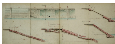
Besançon : projet d'établissement d'un quai au port Rivotte. Dessins de détail des ouvrages [détail : coupes et élévation], 1861.
