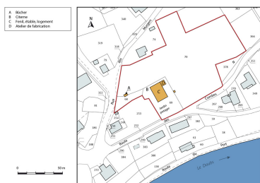
Plan-masse et de situation. Dess. Mathias Papigny IVR43_20162501547NUDA
