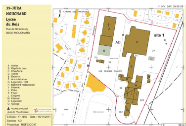
Plan-masse et de situation. Extrait du plan cadastral numérisé 2011, section AD, échelle 1/1 856. Dess. André Céréza IVR43_20113900109NUDA
