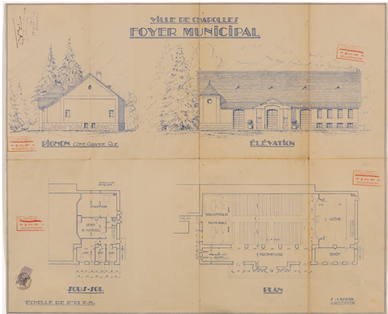
Ville de Charolles. Foyer municipal. Plan d'ensemble [plans et élévations]. S.d. [Visa du 16 avril 1937].
