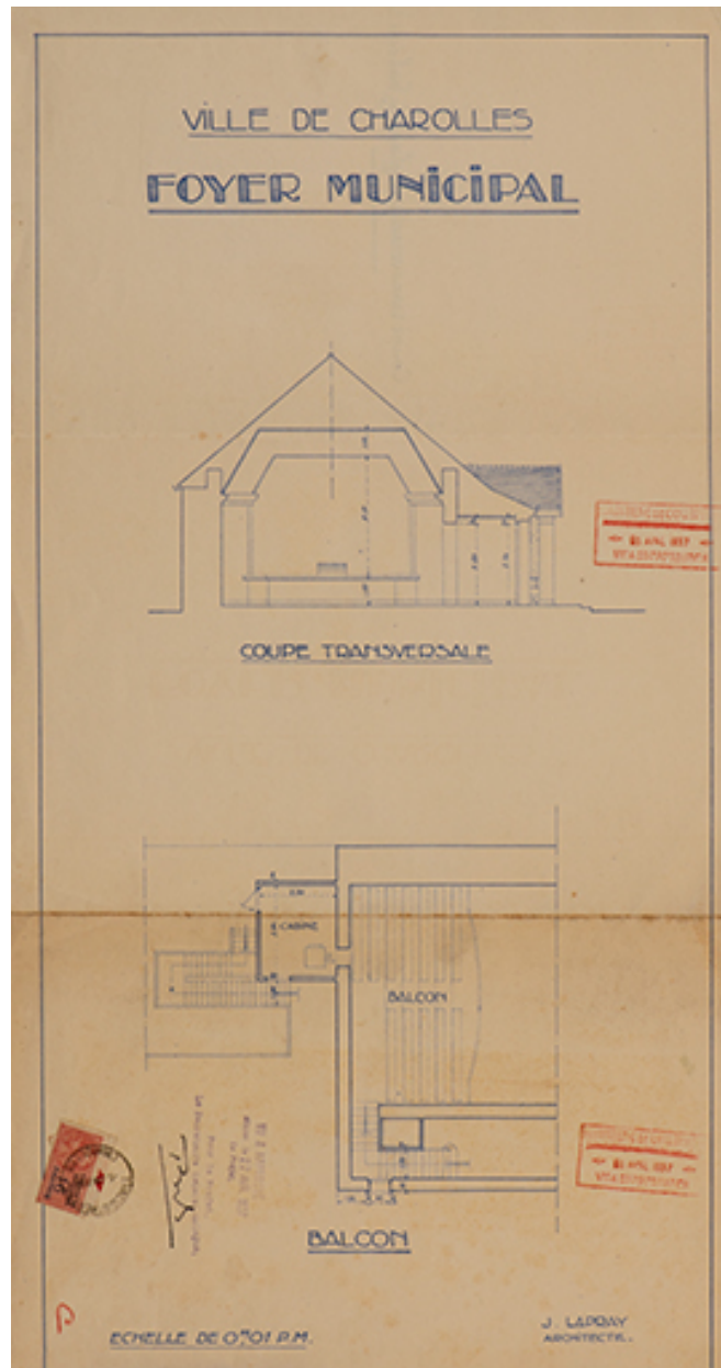
Ville de Charolles. Foyer municipal. Coupe transversale [et] Balcon. S.d. [Visa du 16 avril 1937].
