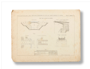
Ponts sur les dérivations de St Jean-de-Losne, Le Châtelet et Seurre. Pont sur l'écluse de Seurre. Plan, coupe et élévation. Phot. Thierry Kuntz IVR26_20172100141NUC4A
