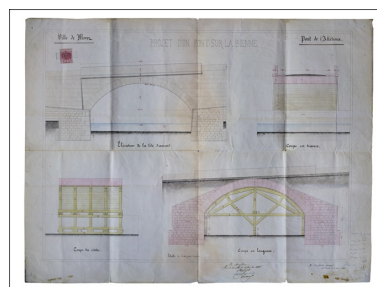
Projet d'un pont sur la Bienne. Pont de l'Affaitieux [élévation amont et coupes], 1866. Phot. Yves Sancey, Phot. Ernest Guillaume IVR43_20103900086NUC2A
