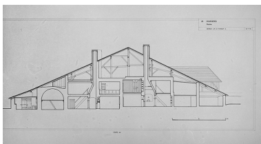
Coupe transversale d'une ferme. Phot. Yves Sancey IVR43_19802500003V
