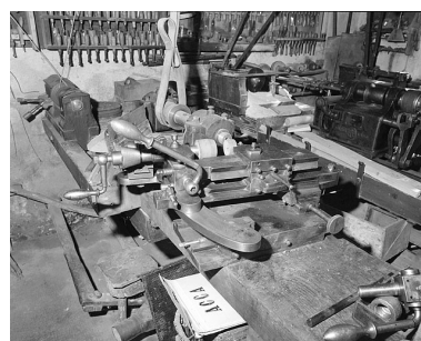
Machine à aplatir. Phot. Jérôme Mongreville IVR43_19963901050X
