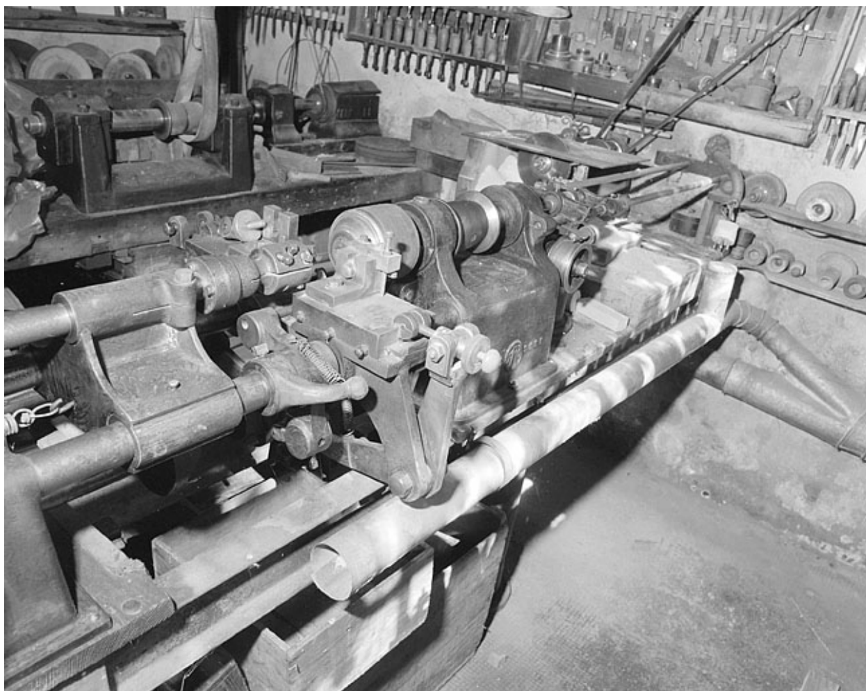
Tour automatique, permettant de travailler la galalithe, datant de 1920 environ.
