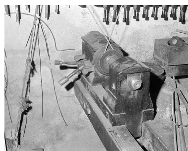
Tour à marchepied : clavier et clés de sélection. Phot. Jérôme Mongreville IVR43_19963901048X
