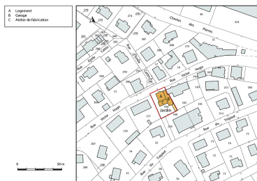
Plan-masse et de situation. Extrait du plan cadastral, 2018, section AF, 1/1 000. Dess. Bertrand Turina IVR43_20182501436NUDA
